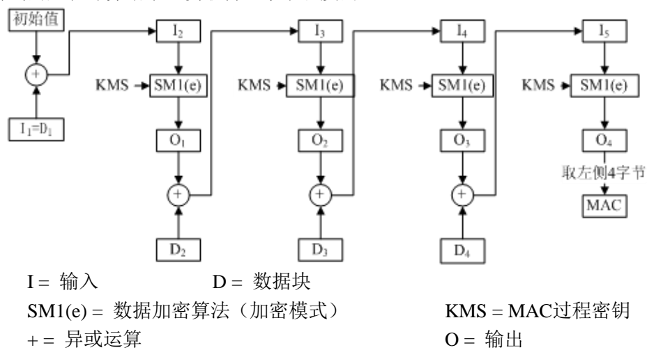
图8 MAC 计算
