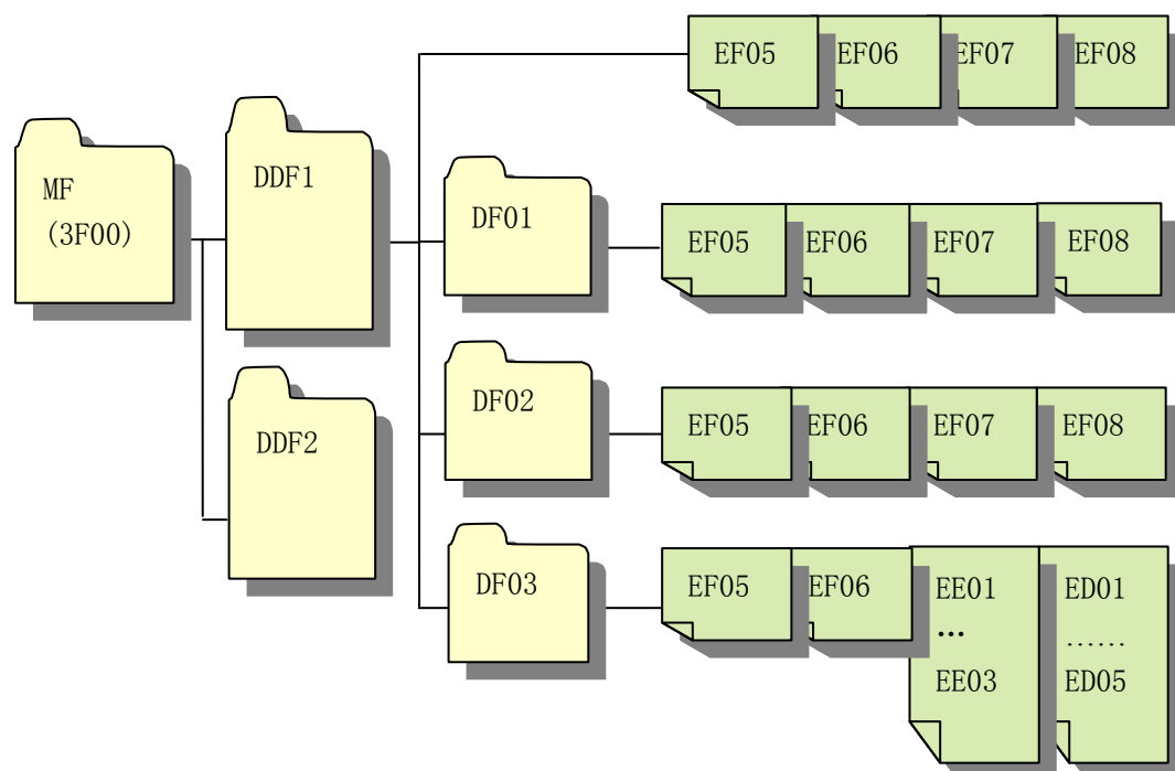
图17 居民健康卡文件结构示意图
